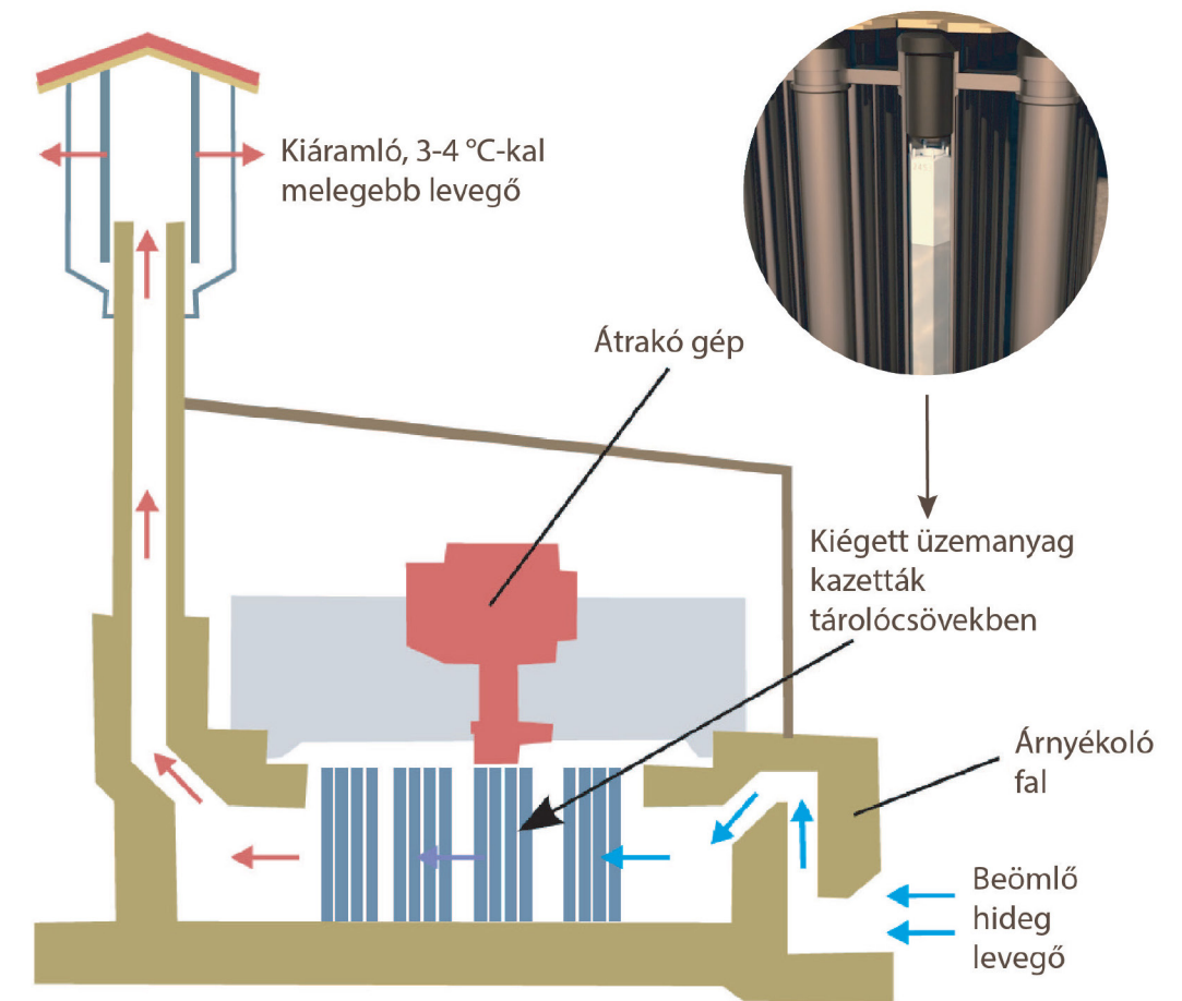
A Kiégett Kazetták Átmeneti Tárolójának keresztmetszete
