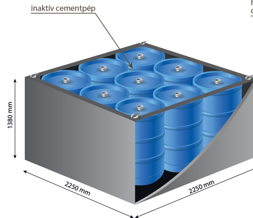
A 3,5-szer kisebb térfogatú KHCS-ban ugyanúgy 1,8 \text{ m}^3 térfogatú radioaktív hulladék helyezhető el, mint a korábbi koncepció szerinti vasbeton konténerben
