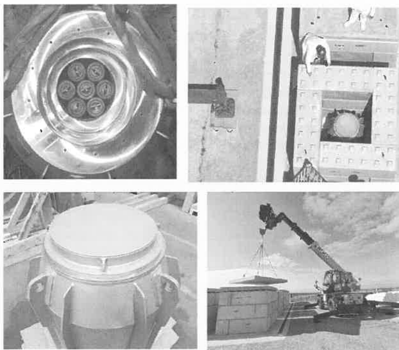
3. ábra: Az RHFT kültéri sugárforrás tároló építménye (jobb felső és alsó kép) és a PRM-2P tároló konténer (bal felső és alsó kép)
