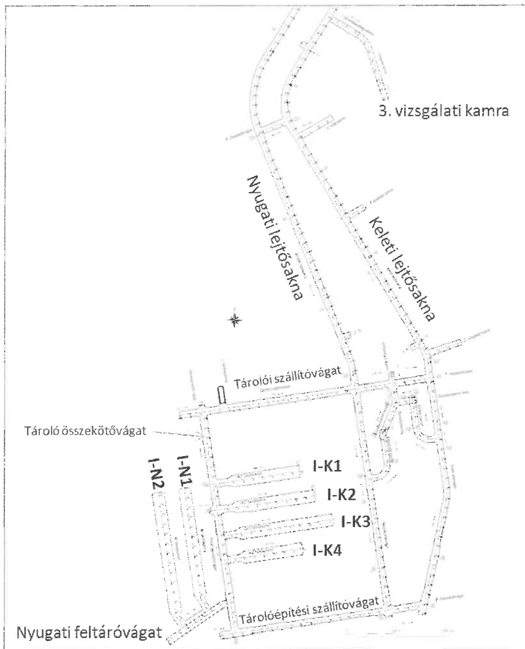
5. ábra: Az I. kamramező vágatrendszere és a 3. vizsgáló kamra
