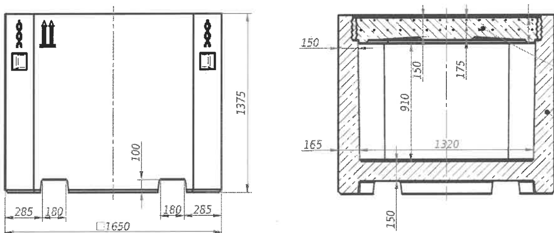
M2. ábra: Paks II kondicionált folyékony hulladékait befogadó kisméretű vasbeton konténerek
