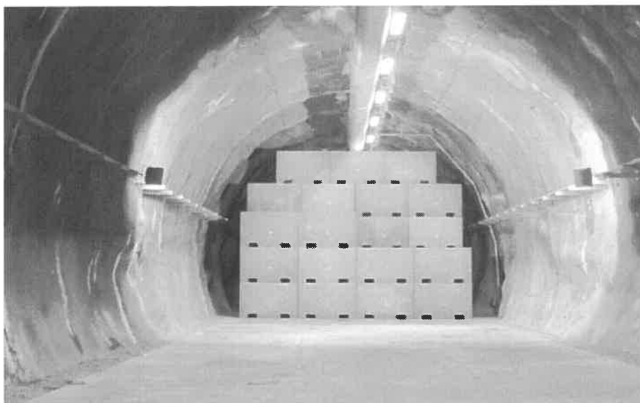
4. ábra: Vasbeton konténerek végleges elhelyezése az I-K1 tárolókamrában
