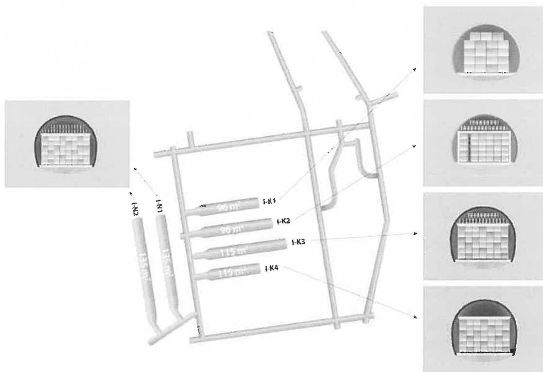
6. ábra: Az I. kamramező kamráiban alkalmazott hulladék elhelyezési rendszer
